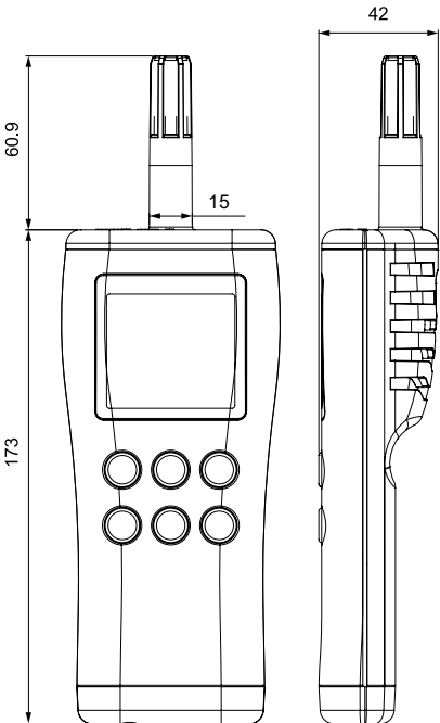
Dimensions CP11
