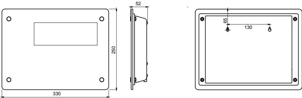
Dimensions CO 2 Display
